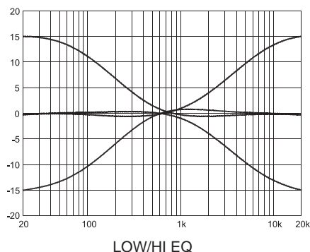
LOW/HI EQ
